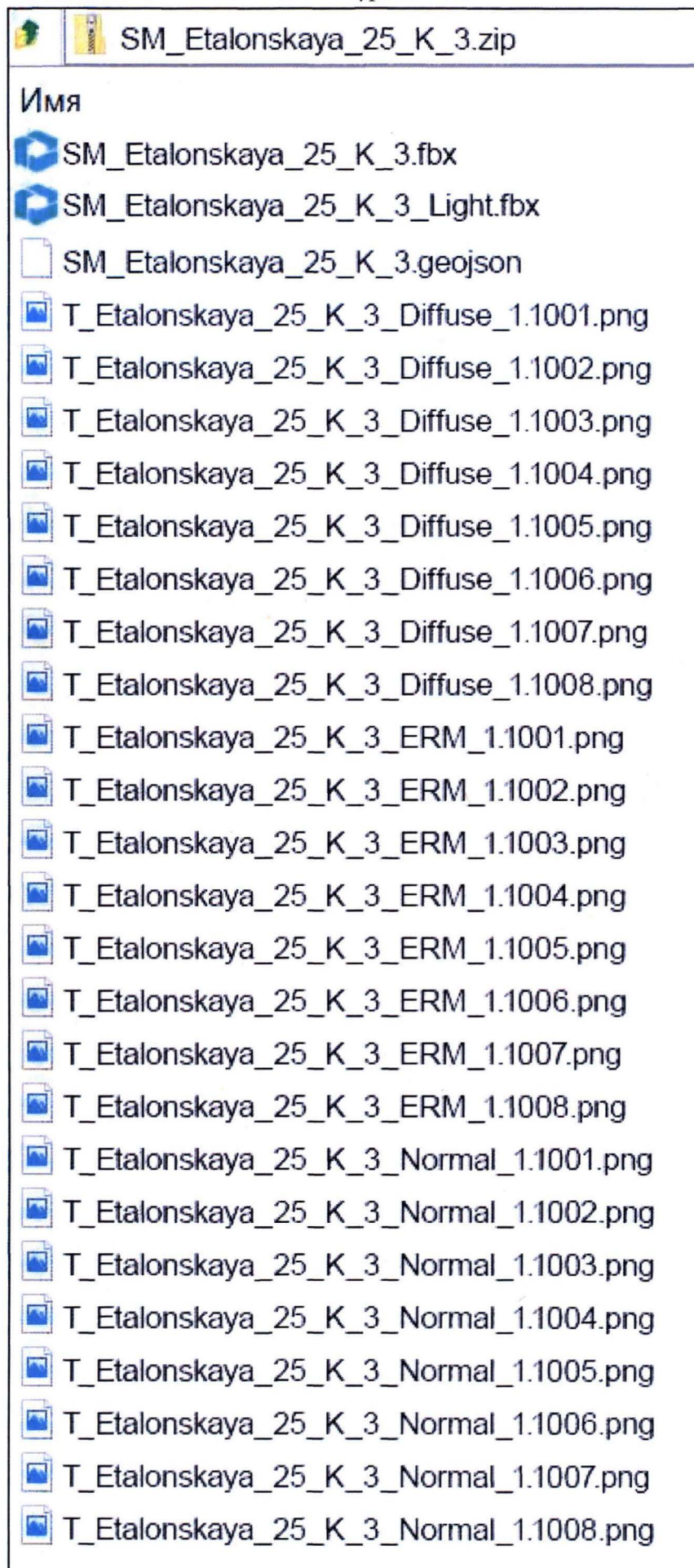
Рис. 2.2. Пример структуры и содержания предоставляемого архива ОКС со световым дизайном фасада
